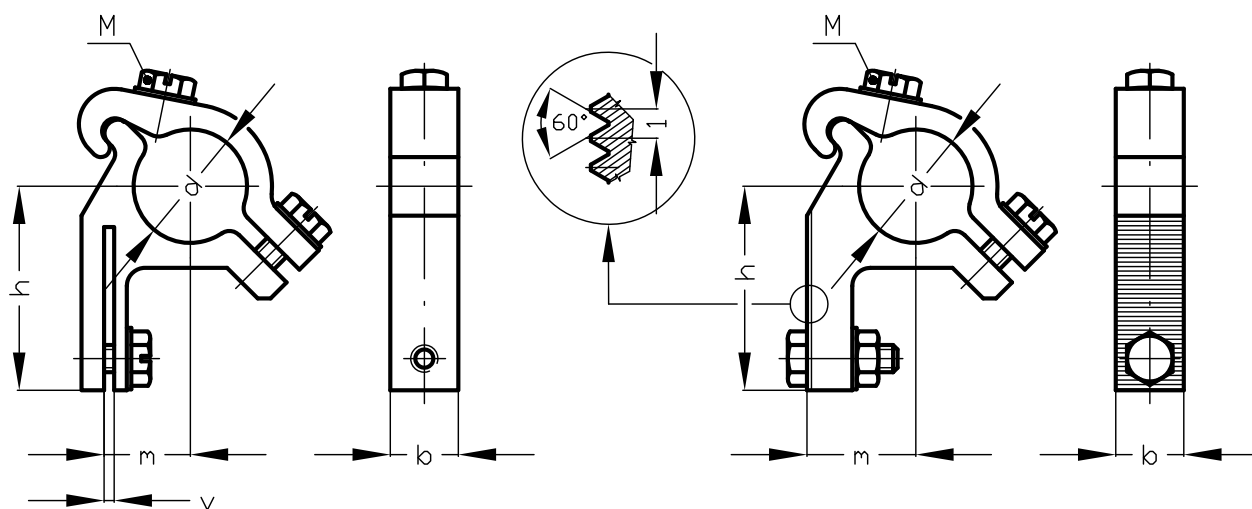
KLEMMSTÜCKE FÜR BÜRSTENHALTER
